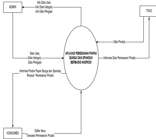
Gambar 2 Diagram Konteks
