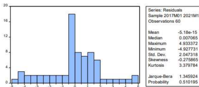
Gambar 1. Uji Normalitas
